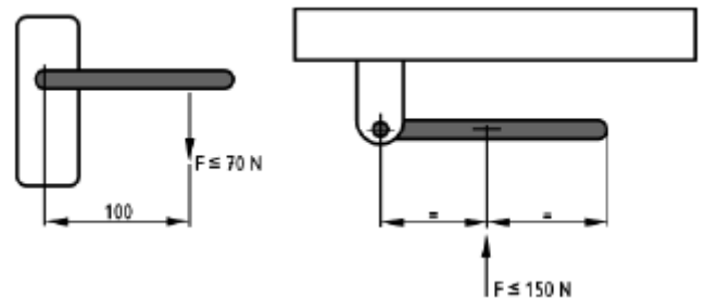
Fermeture de sortie de secours type A
